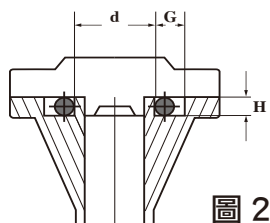
動態使用 (氣體介質) 圖 2
